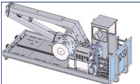
• GT-TM 1750 abgesetzt, in Parkposition
